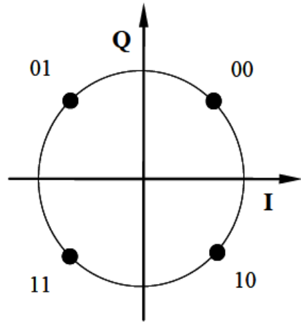
QPSK
