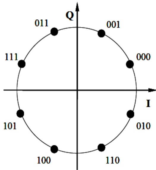
8PSK
